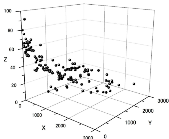
図2. 黒鉛系炭素材料のGG Index (X, Y, Zのみ).
